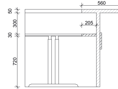
SNITT D:D
