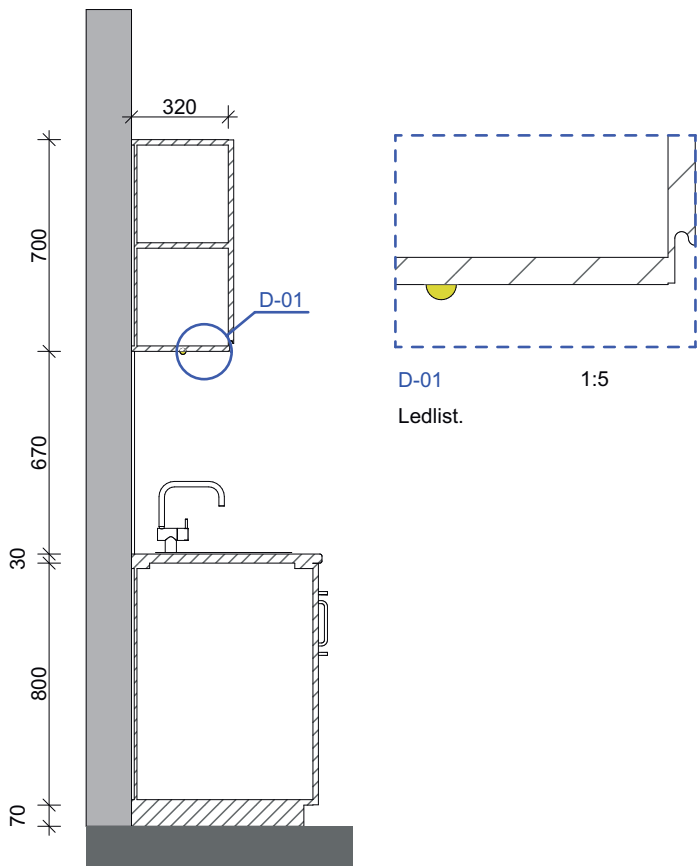
SNITT B:B
