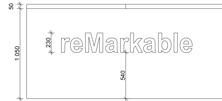
OPPRISS A:A
