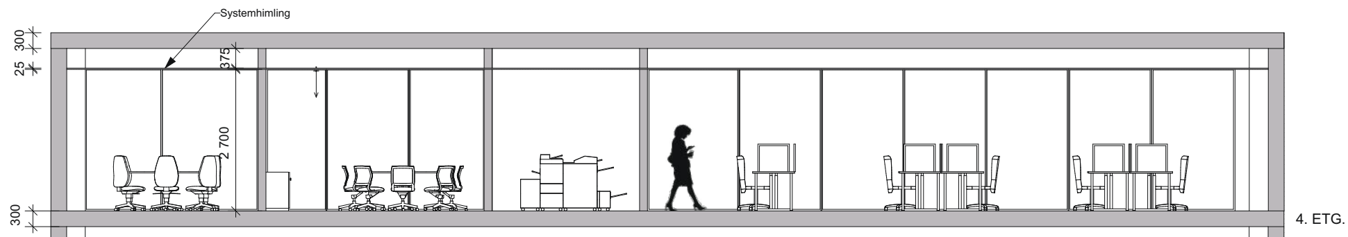
SNITT D:D
