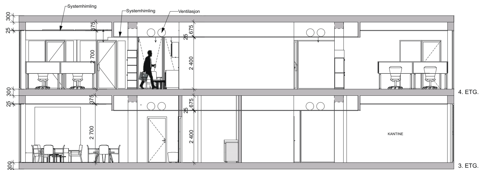
SNITT A:A
