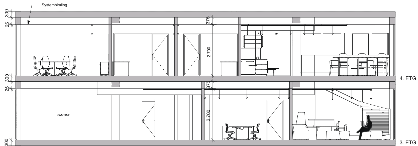
SNITT C:C
