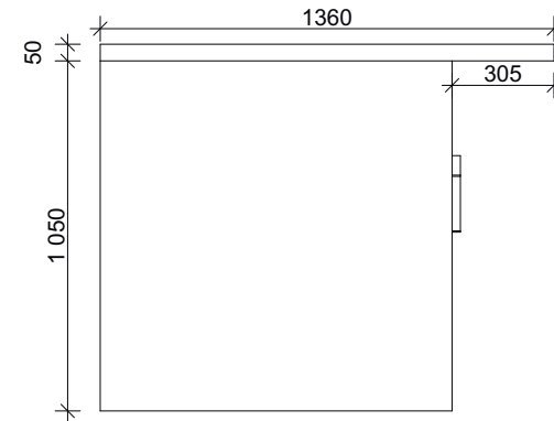
OPPRISS C:C
