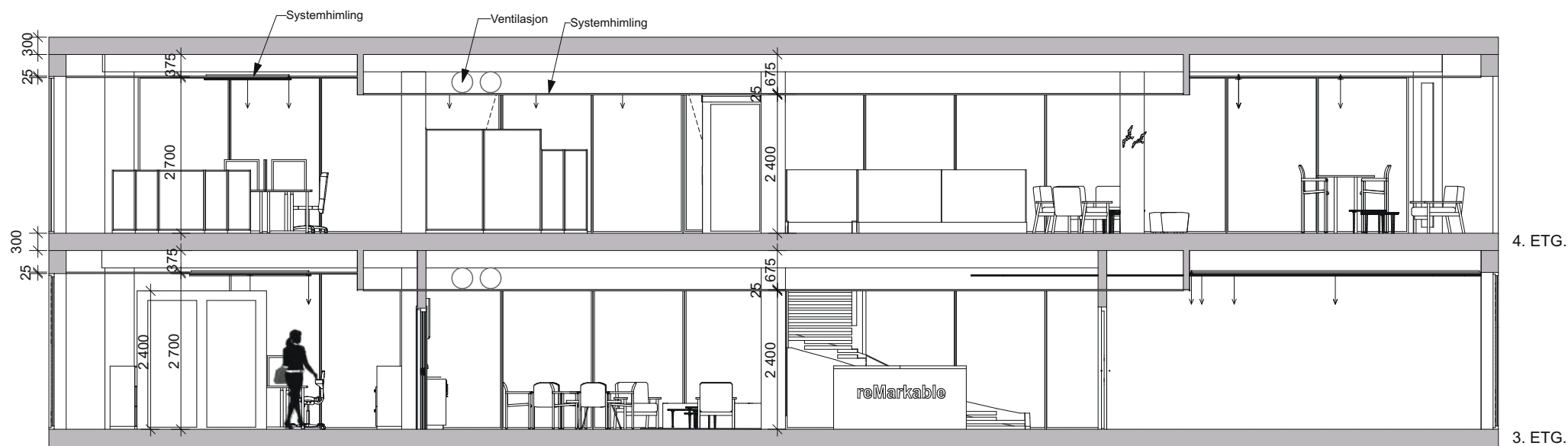
SNITT B:B
