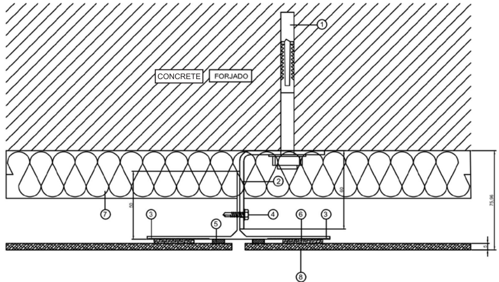
HORIZONTAL SECTION/ SECCIÓN HORIZONTAL
