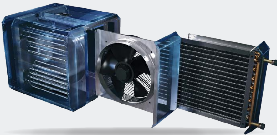
Opbouw binnenunit QSE: warmtewisselaar voor warmtepomp + ventilator + elektrische booster
