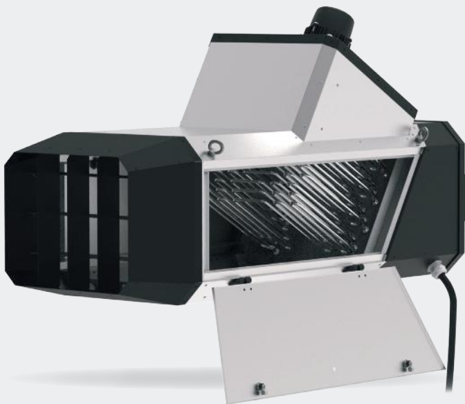
De DX-EH is eenvoudig toegankelijk voor reiniging via het zijluik.
