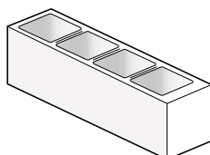
Pustak Fini Lungo (PFL) wymiar: 83,5x19,5x20 cm waga: ~37 kg ilość na palecie: 30 szt.
