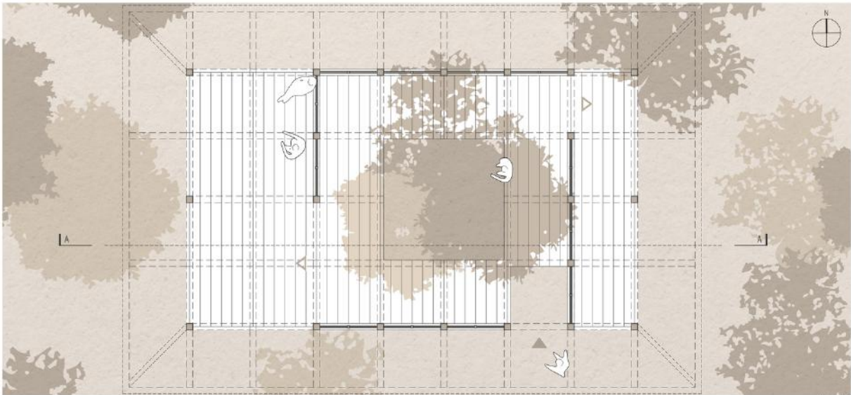
Rzut, 1:50
