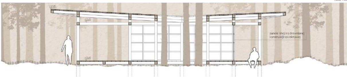
Przekrój, 1:50
