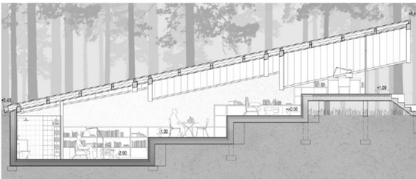
Przekrój
