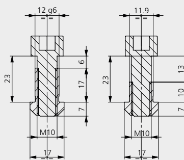
► T-SLOT 12 46204103
