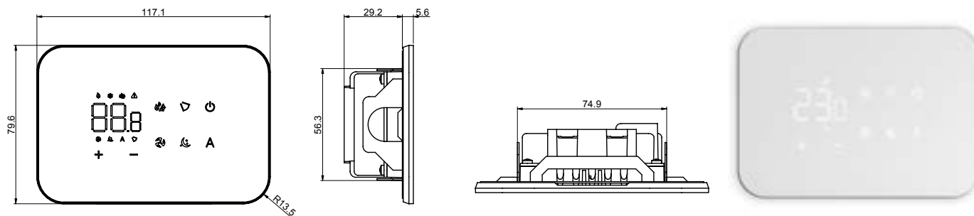
SMART M7-Touch control panel part n° 3C0025829B
