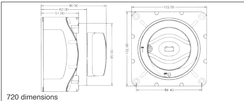
720 dimensions
