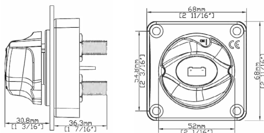
701-PM dimensions
