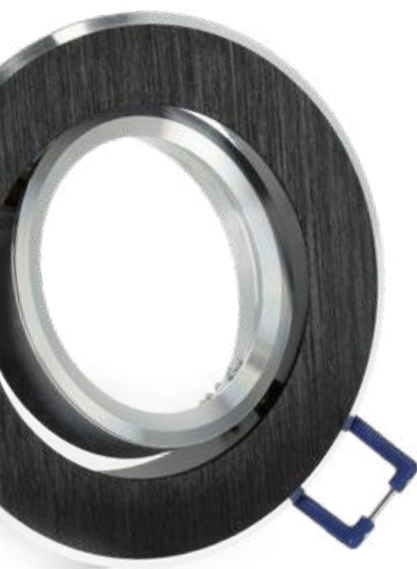
Pierścień ozdobny / Downlight ring OH29 Kobi mat czarny / matt black | IP20 | wymiary / size: Ø 8,5 x 2,7 cm 002078 | EAN: 5902201305463
