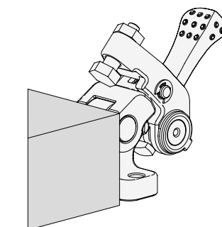
1. Posizione staffa prima del bloccaggio
