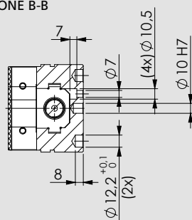
SEZIONE B-B
