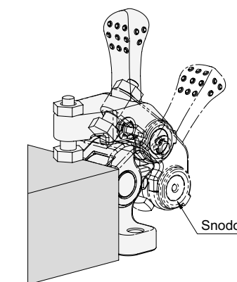
2. Posizione inizio bloccaggio
