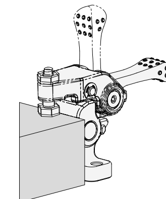
3. Bloccaggio: Spingere la leva verso il basso per bloccare il pezzo.
