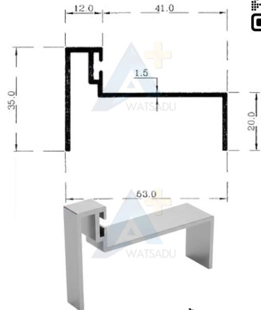
NO. 4265 บังใบ 2 นิ้ว
