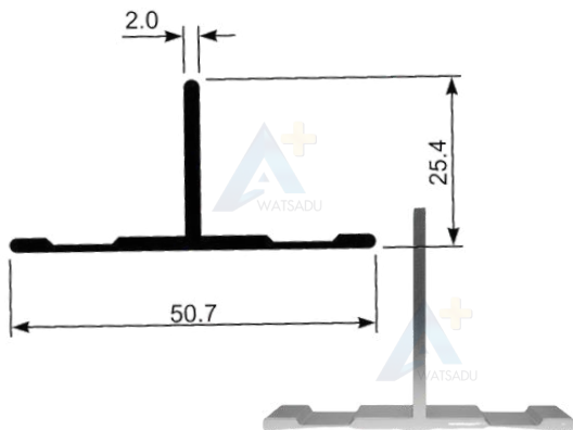
NO. 1683 ตัวที 2 นิ้ว ยาว 6 เมตร
