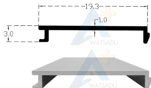
NO.6116 ฝาปิดตัวเล็ก
