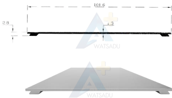
NO.9037 ฝาแฉีกสัน
