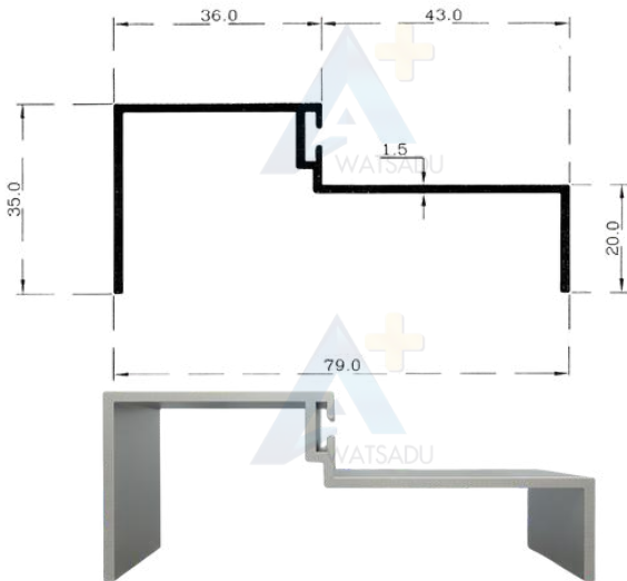
NO.4264 บังใบ 3 นิ้ว
