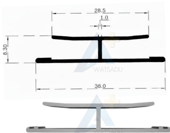
NO. 1684 ตัวไอเล็ก
