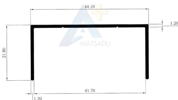
NO.4260 รางยู 40 มม.
