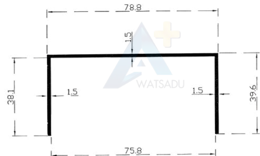
NO.4259 รางยู75 อะลูมิเนียม
