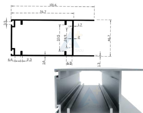
NO. PT291 กรอบบานประตู ห้องเย็น ห้องคลีนรูม
