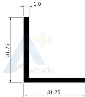
NO.179 จากอะลูมิเนียม 1.2"X1.2"
