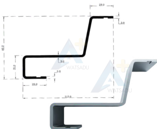
NO.4250 เฟรมสวิง 3 นิ้ว
