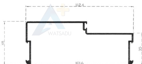
NO.6120 จากแอล ไร้รีเวท
