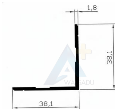
NO.918 จากหนา จากลาย 1"X1"
