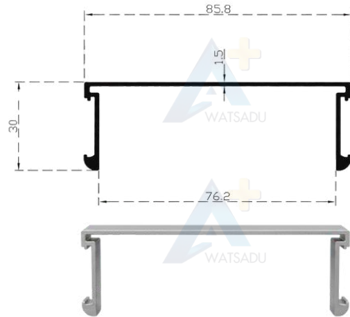
NO.6119 ตัวยู 3 นิ้ว ไร้รีเวท
