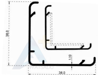
NO.PT-95 จากอะลูมิเนียม 1.5"X1.5" หนา 1.10 มม. ยาว 6 เมตร แบบ 2 ชั้น
