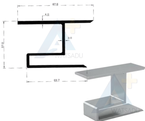
NO. 1687 กรอบไคด์ 2 นิ้ว
