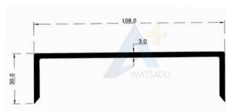
NO.1691 รางยู 100 อะลูมิเนียม
