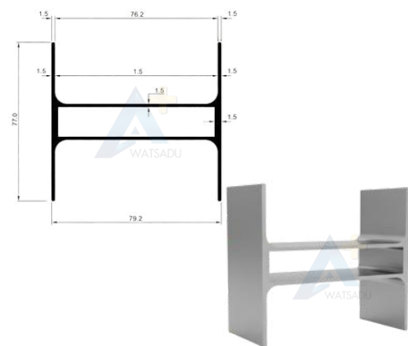
NO.1701 ตัวเอก 3 ชั้น
