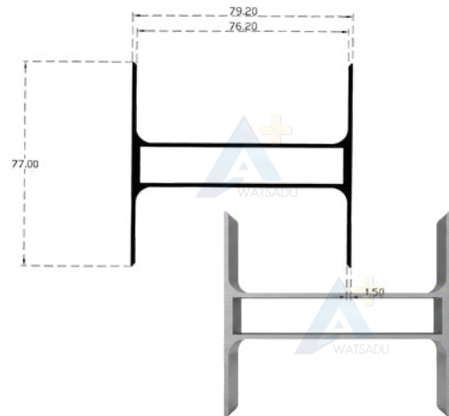
NO. 6125 ตัวเอก 3" มีรูไร้รีเวท
