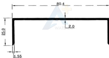
NO.1690 รางยู 75 อะลูมิเนียม
