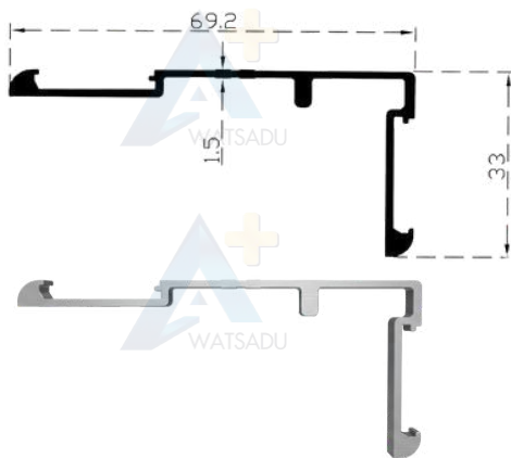
NO.6120 จากแอล ไร้รีเวท
