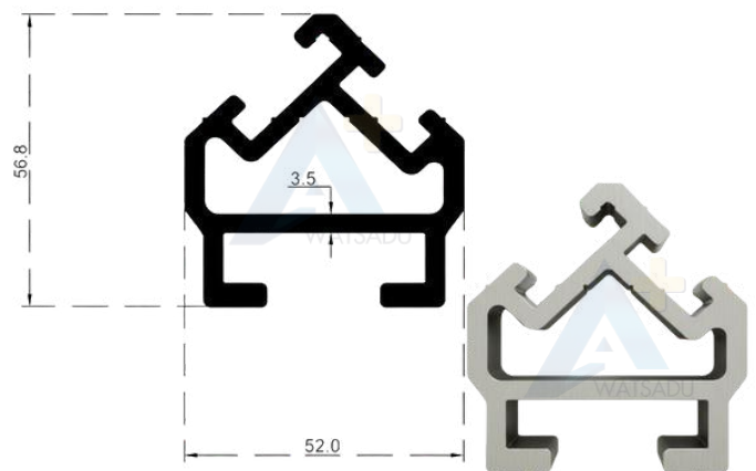
NO. 6009 คานล่อง 52.0 มิล มุงกฤษ
