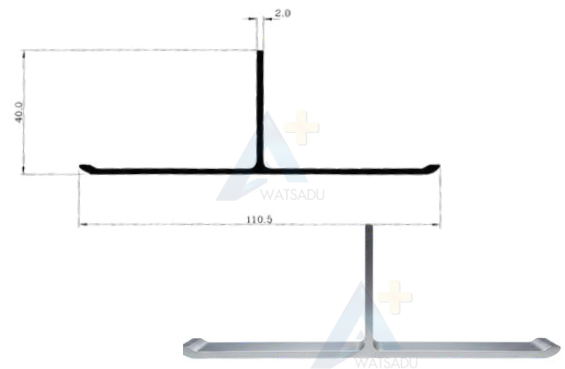
NO.26 ตัวที 2 นิ้ว ยาว 6 เมตร
