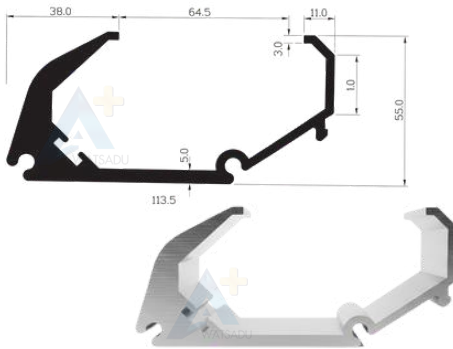
NO. 1746 รางก้ามปู
