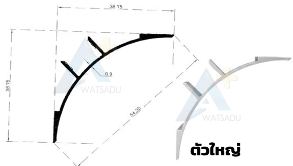
NO.1113 จากตบโค้ง ยาว 6 เมตร
