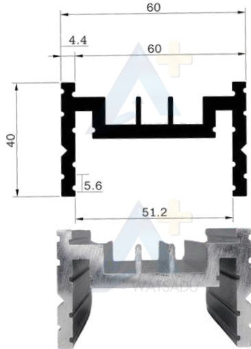
NO. PT 91 รางฮีตเตอร์ ยาว 6 เมตร
