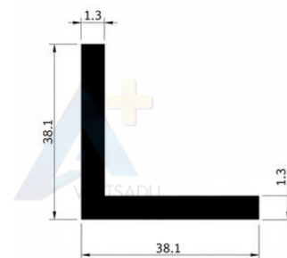
NO.191 จากบางอะลูมิเนียม 1"X1"
