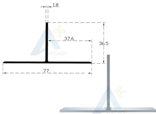
NO.6117 ตัวที 3 นิ้ว ไร้รีเวท
