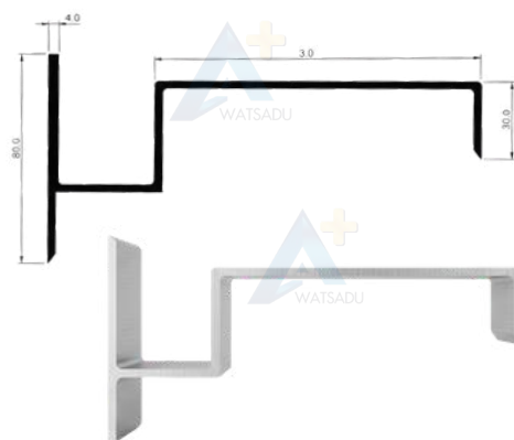
NO. 1686 กรอบไกด 6 นิ้ว
