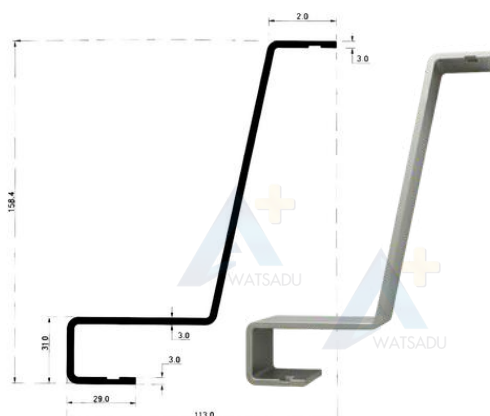
NO.4252 เฟรมสวิง 6 นิ้ว
