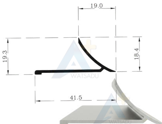
NO. 1684 ตัวไอเล็ก
