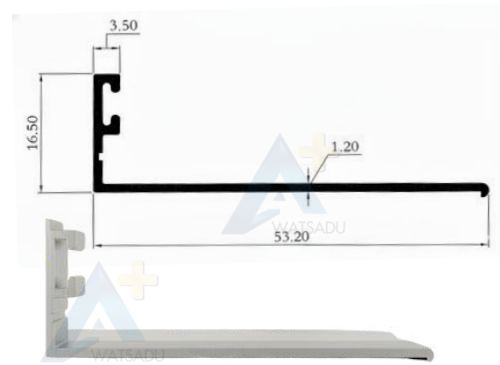
NO.4267 ฉากบังใบ
