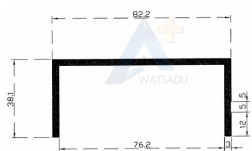
NO. PT - 271 รางยู75
