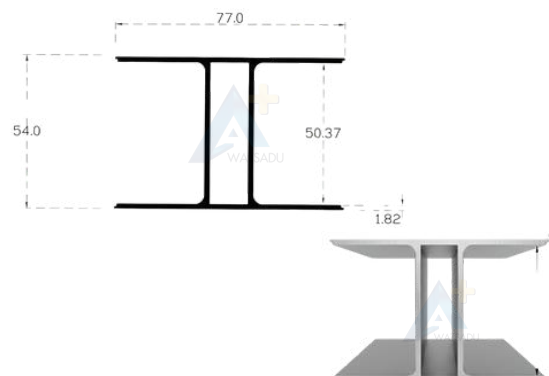
NO.6126 ตัวเอก 2" มีรูไว้รีเวท
