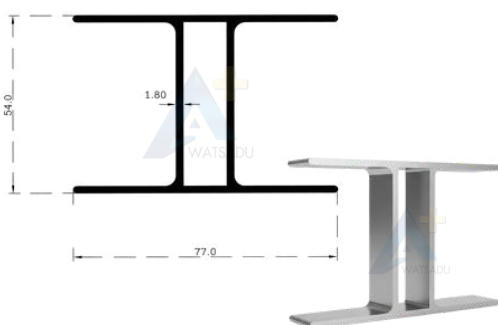
NO.4266 ตัวเอก 2 ชั้น
