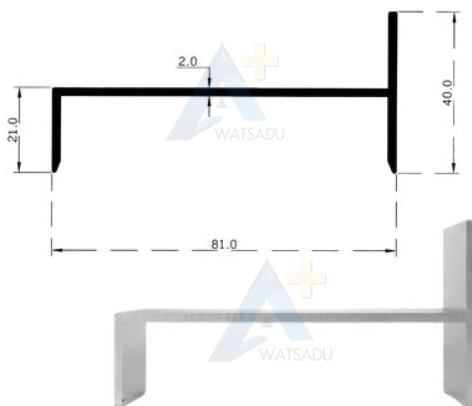
NO. 4263 ตัวเจ 2 นิ้ว
