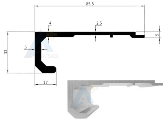
NO.14915 รางตัวเจ 3 นิ้ว
