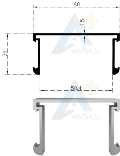
NO.6118 ตัวยู 2 นิ้ว ไร้รีเวท
