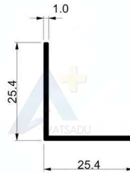
NO.166 จากอะลูมิเนียม 1"X1"
