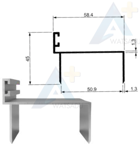
NO.PT 233 รางยูบังใบ 2 นิ้ว
