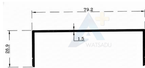
NO.4257 รางยู75 อะลูมิเนียม
