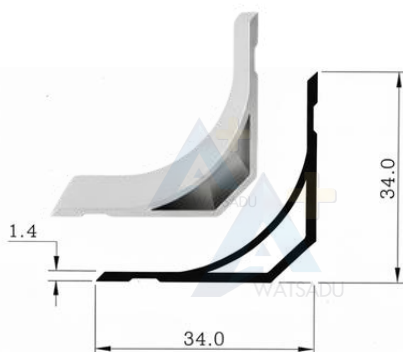
NO.1682 จากตบโค้งขึ้นเดียว ยาว 6 เมตร
