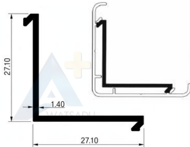
NO.PT-94 จากอะลูมิเนียม 1.5"X1.5" หนา 1.4 มม. ยาว 6 เมตร แบบ 2 ชั้น
