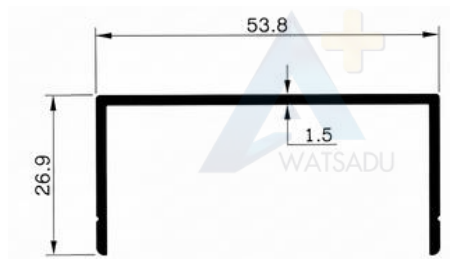
NO.4256 รางยู50 อะลูมิเนียม
