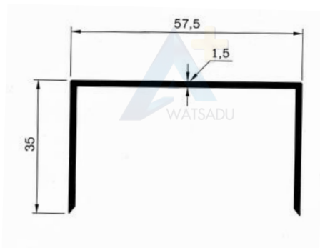
NO. PT-145 รางยู50 อะลูมิเนียม
