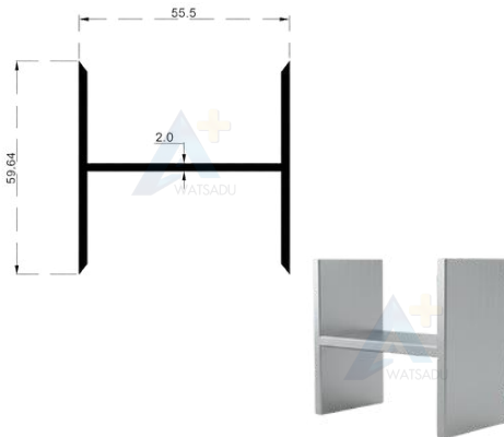
NO.1693 ตัวเอก 2 ชั้น
