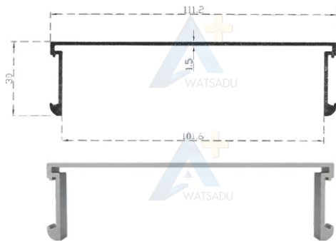
NO. 6124 ตัวยู 4 นิ้ว ไร้รีเวท
