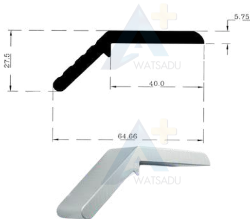
NO. 6008 โถงด้านล่าง จากห้องเย็น 45 องศา
