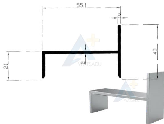
NO. PT 78 ตัวเจ 2 นิ้ว
