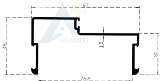
NO. 6121 บังใบ 2 นิ้ว ไร้รีเวท
