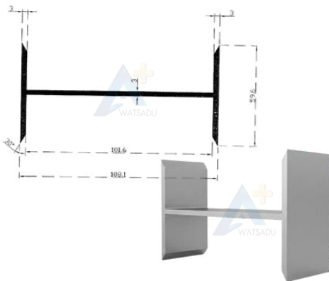
NO.1695 ตัวเอก 4 ชั้น
