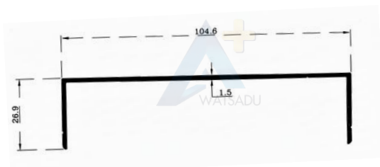
NO. 4258 รางยู 100 อะลูมิเนียม
