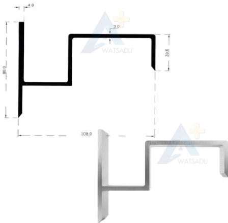
NO. 1688 กรอบไคด์ 4 นิ้ว
