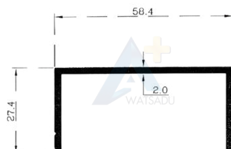
NO.4253 รางยู 50 อะลูมิเนียม
