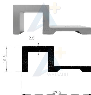
NO. 4262 ครอบฮีตเตอร์
