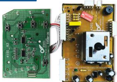
KIT PLACA POTÊNCIA COMPAT. LTC10 V2 - 70201296 - BIVOLT
