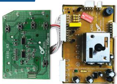
KIT PLACA POTÊNCIA COMPAT. LT13B A99035102 A99035120 A99035179 BIVOLT
