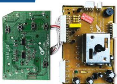
KIT PLACA POTÊNCIA COMPAT. LES15 / L W20 A13611012 - BIVOLT
