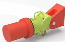
Abrazadera hidráulica de cilindro SB40 7.8in/200mm 5000174 Compatible con Sandvik DD421/i y DD422/i
