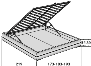
Misura interne vano contenitore: cm. 159/169/179 x 200 x 24h
