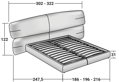
misura testata: 302 per materassi 170 / 180 322 per materassi 200
