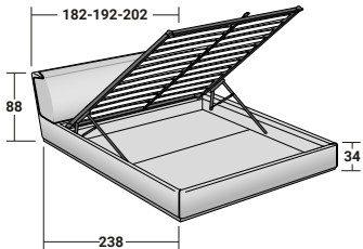
Misure interne vano contenitore: cm. 159/169/179x200x16,5 h
