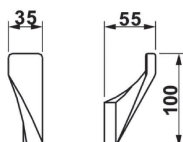
Belbagno Item Description AM-G-2738 Robe Hook
