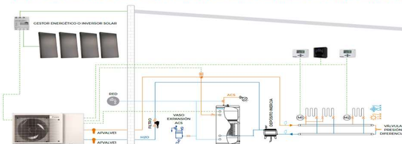
Ejemplo Daikin Altherma 3 Monobloc con depósito para ACS y suelo radiante, complementado con energía solar fotovoltaica
