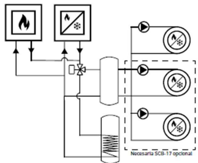
Solucion climatización y ACS híbrida con caldera de gas o gasóleo
