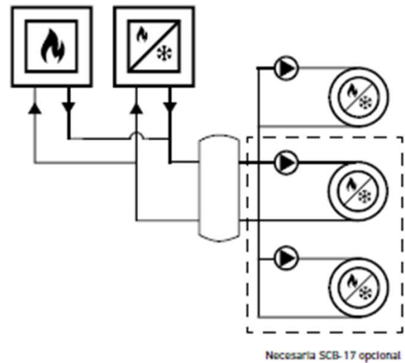
Solucion climatización y ACS híbrida con caldera de gas o gasóleo
