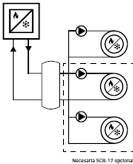
Solucion climatización y ACS
