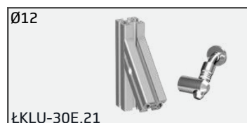
ŁKLU-30E.21 łącznik kątowy lewy, uniwersalny 30E, Ø12
