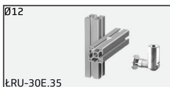
Łącznik równoległy uniwersalny 30E, Ø12
