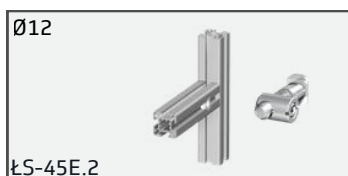
Łącznik standardowy 45E, Ø12
