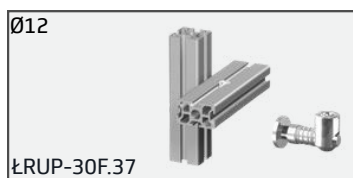
Łącznik równoległy uniwersalny, poprzeczny 30/50-F, Ø12
