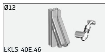
Łącznik kątowy lewy, standardowy 40E, Ø12
