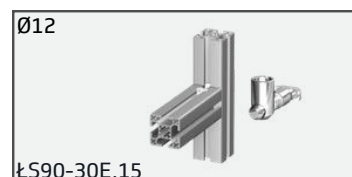
ŁS90-30E.15 łącznik standardowy 90°, 30E, Ø12
