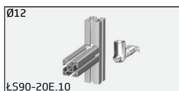
ŁS90-20E.10 łącznik standardowy 90°, 20E, Ø12
