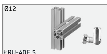
ŁRU-40E.5 Łącznik równoległy uniwersalny 40E Ø12
