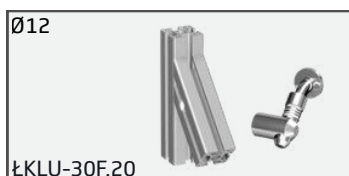
ŁKLU-30F.20 łącznik kątowy lewy, uniwersalny 30F, Ø12
