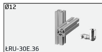
Łącznik równoległy, standardowy 30E, Ø12
