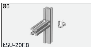
ŁSU-20F.8 łącznik standardowy, uniwersalny 20F, Ø6
