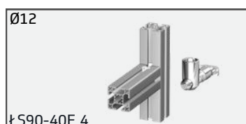
ŁS90-40E.4 Łącznik standardowy 90°, 40E, Ø12
