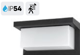
Kinkiet ogrodowy / Garden wall lamp LED LENTERO 12W LX IP54 LED2B czarny / black | IK06 | IP54 | 110° | 12W | 840 lm | wymiały / size: 26 x 12,5 x 12,5 cm 4000K: 003705 | EAN: 5902201391411
