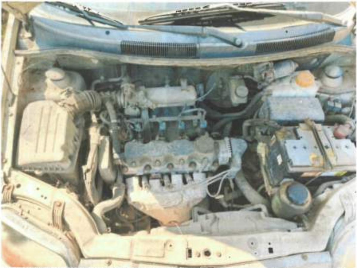
Fotografía 21. Habitáculo del motor, presenta varias partes con corrosión, laterales y centro.
