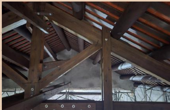
修復中的禮拜堂屋架與椽條。
