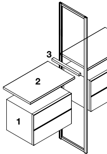
Accostamento fianco/divisione Telaio 1 Modulo o moduli cassetiera 2 Top cassetiera 3 Traverso cassetiera (tipo C) a due cassetteiere affiancate
