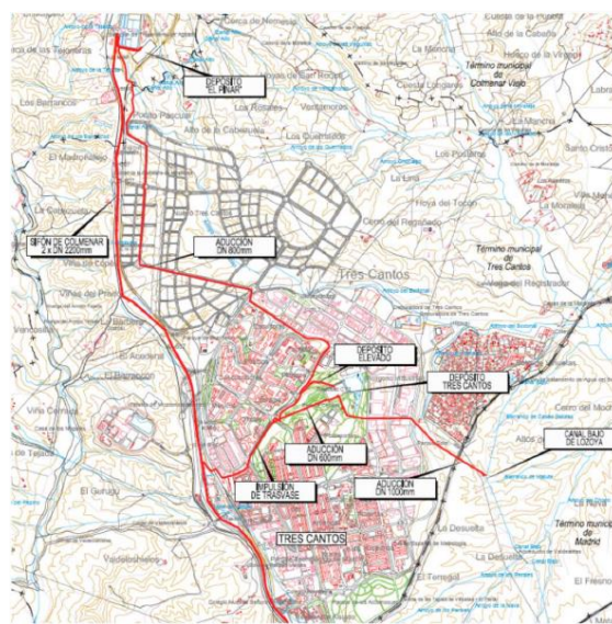
Figura 20: Elementos de la red de abastecimiento de agua de Tres Cantos. Fuente: Canal Isabel II.
