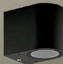
K1201N. Aluminio. 1×GU10. 10×7×8cm. Negro. IP54.
