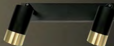
U2132. 2×GU10. 25×6cm. Negro+Dorado.
