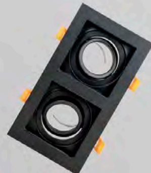
EM7002N. 2xGU10, 100x185mm. Metal. Orientable. Negro.
