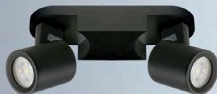
U1302N. Aluminio. 2×GU10. 22×7×12,5cm. Negro.
