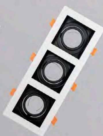
EM7003B+N. 3xGU10, 100x270mm. Metal. Orientable. Blanco + Negro.
