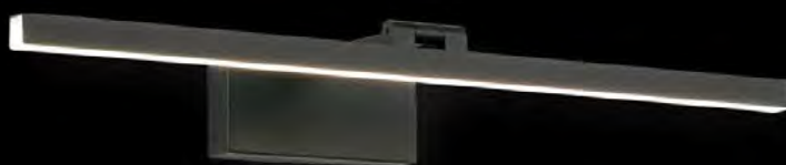
L2316N. LED 16W 3000K. 59×8×18cm. Negro.
