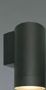
K1401N. Aluminio. 1×GU10. 12×6,5×9cm. Negro. IP54.
