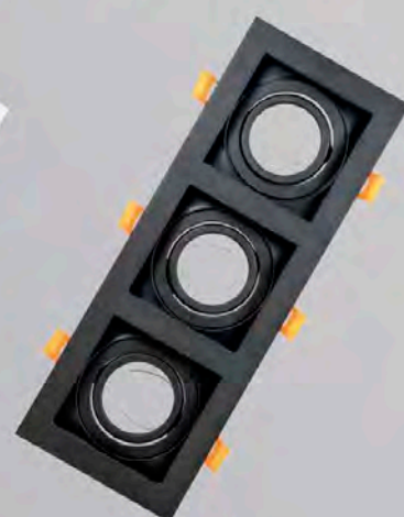
EM7003N. 3xGU10, 100x270mm. Metal. Orientable. Negro.
