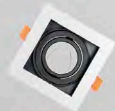
EM7000B+N. 1xGU10, 100x100mm. Metal. Orientable. Blanco + Negro.
