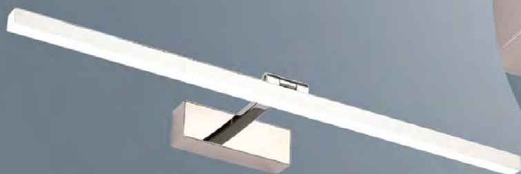
L0216. LED 16W 3000K. 59×8×18cm. Cromo.
