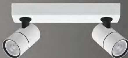
U1322B. Aluminio. 2×GU10. 25×6×16cm. Blanco.
