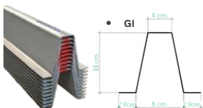
แปโอเมกา Purlin Omega
