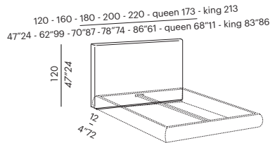
esempio di composizione - sketch of configuration
