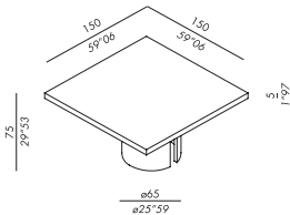
tavolo pranzo 150-TP - dining table 150-TP
