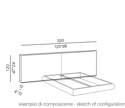
esempio di composizione - sketch of configuration
