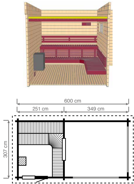
2 Elegance schuiframen, 1 sauna deur en 1 sauna venster verticaal en 1 horizontaal
