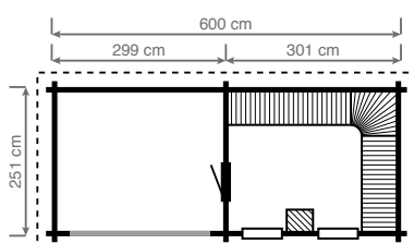
1 Elegance schuifraam, 1 sauna deur en 2 sauna vensters verticaal
