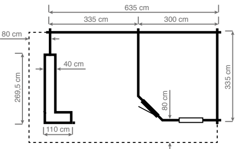
1 enkele matglasdeur en 1 raam met matglas folie
