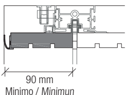
Fascia di tamponamento iniziale Initial filler
