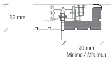
Fascia di tamponamento terminale Terminal filler
