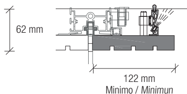
Fascia di tamponamento terminale con LED Terminale filler with LED
