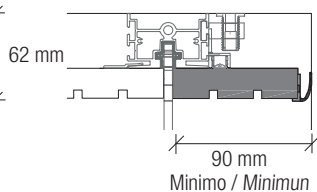
Fascia di tamponamento terminale Terminal filler
