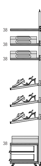
SEZIONE D-D / SECTION D-D
