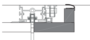
Fascia di tamponamento terminale Terminal filler
