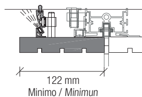
Fascia di tamponamento iniziale con LED Initial filler with LED
