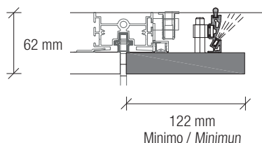
Fascia di tamponamento terminale con LED Terminale filler with LED
