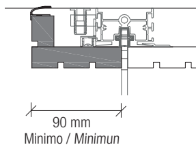
Fascia di tamponamento iniziale Initial filler
