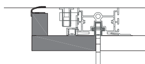
Fascia di tamponamento iniziale Initail filler
