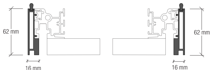
Chiusura verticale INIZIALE INITIAL side closure
