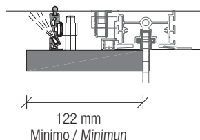
Fascia di tamponamento iniziale con LED Initial filler with LED
