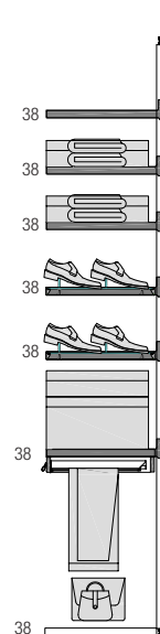
SEZIONE F-F / SECTION F-F
