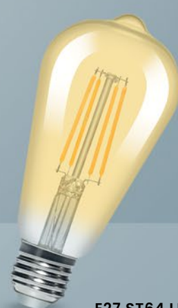
E27 ST64 LED 8w 800 lm dimerizable 2700K Ámbar
