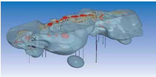
Modèle géologique 3D du projet Montauban. / 3D geological model of the Montauban Project.
