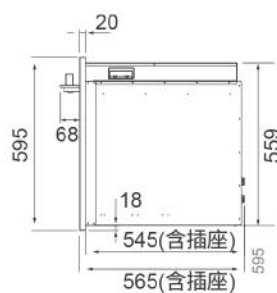
側視圖
