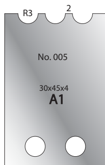
Cutter: 005H00005 Limiter: 006H00005
