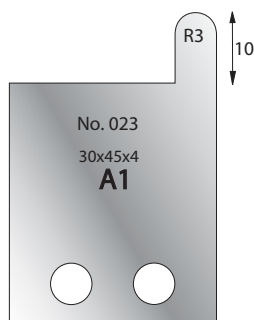
Cutter: 005H00023 Limiter: 006H00023
