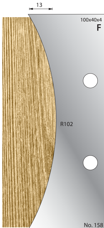
Cutter: 003H00158 Limiter: 004H00158
