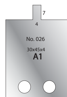
Cutter: 005H00026 Limiter: 006H00026
