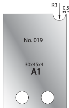
Cutter: 005H00019 Limiter: 006H00019
