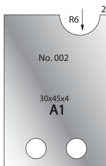
Cutter: 005H00002 Limiter: 006H00002
