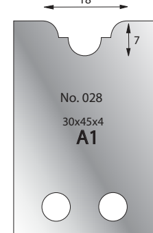
Cutter: 005H00028 Limiter: 006H00028
