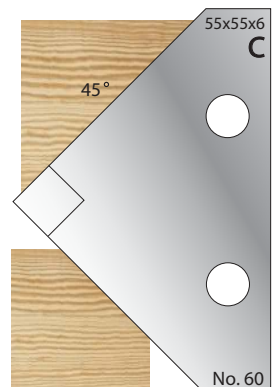
Cutter: 003H00060 Limiter: 004H00060
