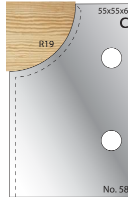
Cutter: 003H00058 Limiter: 004H00058
