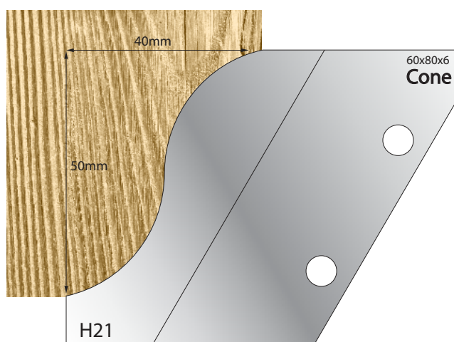
Cutter: 003H00H21 Limiter: 004H00H21
