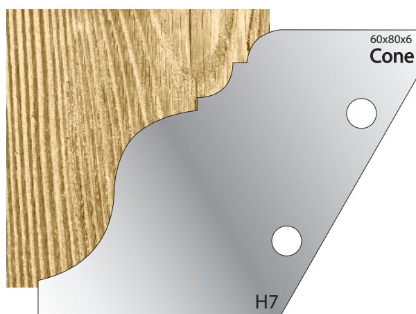
Cutter: 003H000H7 Limiter: 004H000H7
