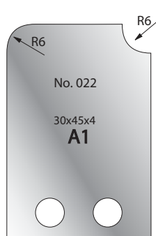
Cutter: 005H00022 Limiter: 006H00022
