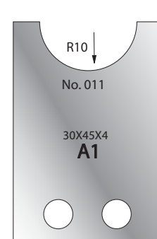
Cutter: 005H00011 Limiter: 006H00011
