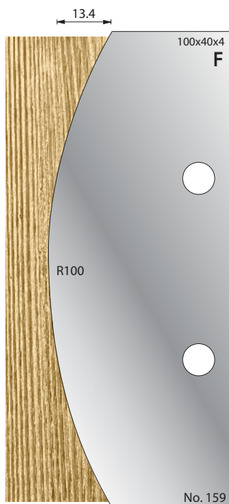
Cutter: 003H00159 Limiter: 004H00159
