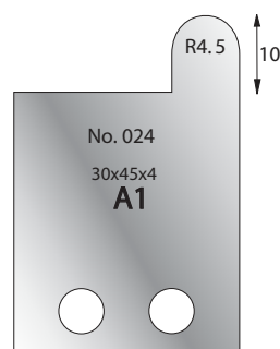
Cutter: 005H00024 Limiter: 006H00024
