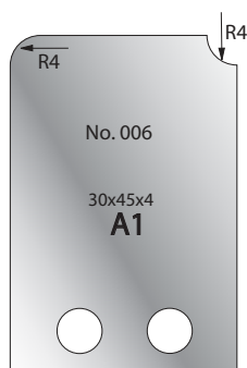
Cutter: 005H00006 Limiter: 006H00006
