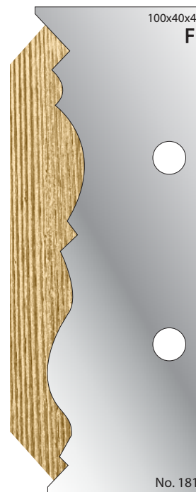
Cutter: 003H00181 Limiter: 004H00181
