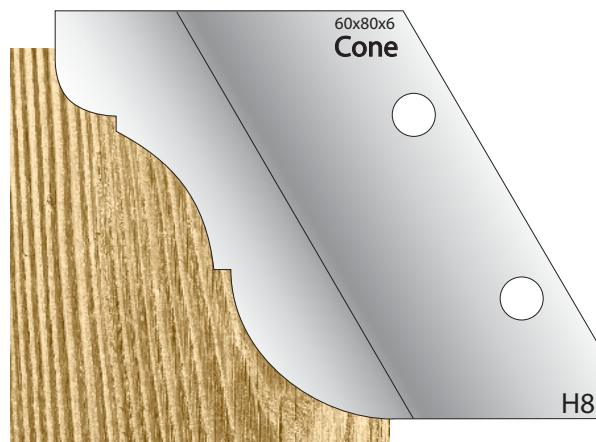
Cutter: 003H000H8 Limiter: 004H000H8
