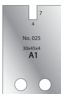
Cutter: 005H00025 Limiter: 006H00025
