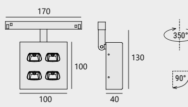
48V track/szynoprzewód 48V
