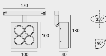
48V track/szynoprzewód 48V
