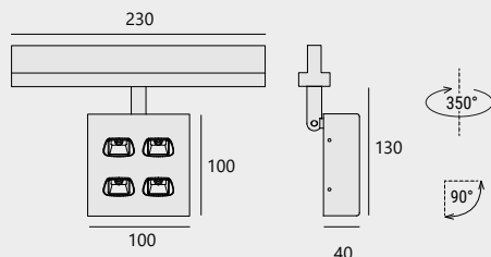
track 230V/szynoprzewód 230V
