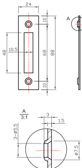
CONTRAFRONTAL
