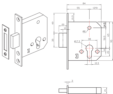
CERRADURA
