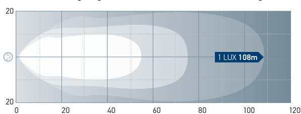
Module 70 Gen 5 Long Range
