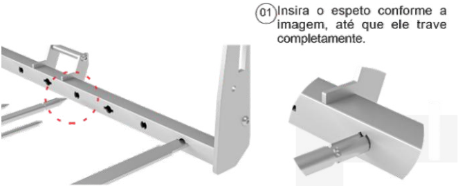
Figura 5 - Encaixe dos espetos.
