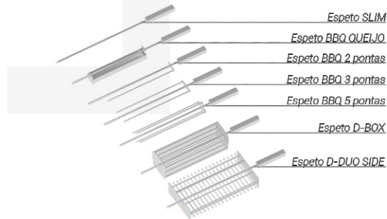
Figura 4 – Espetos.
