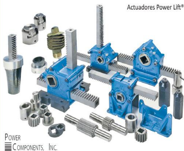
Actuadores Power Lift®
