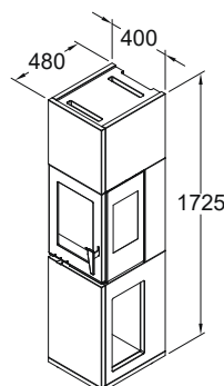
VisionLine i40-3 Elementpeis (med sideglass)
