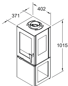
VisionLine s40-3 (med sideglass)
