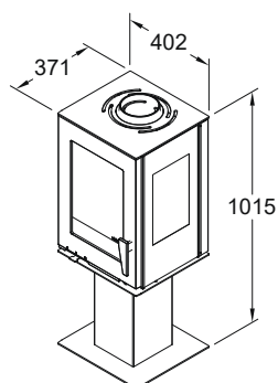
VisionLine s40-3 Pidestall (med sideglass)
