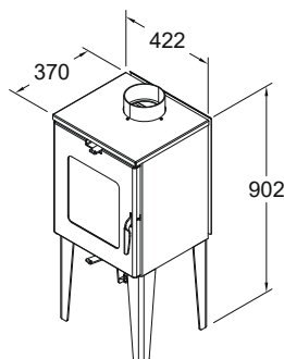
VisionLine s25-1 (uten sideglass)
