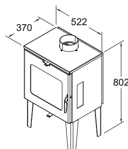
VisionLine s35-3 (med sideglass)
