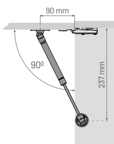
Vista Lateral: Apertura 90°
