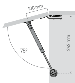
Vista Lateral: Apertura 75°
