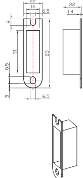
EMBELLECEDOR
