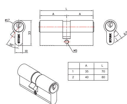
CILINDRO LLAVE/LLAVE
