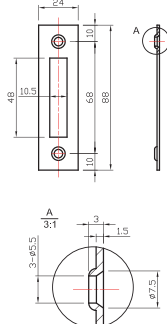
CONTRAFRONTAL
