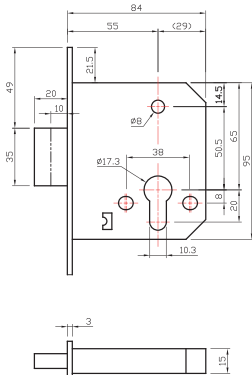
CERRADURA
