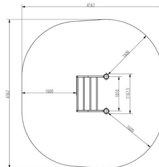
Felülnézet
