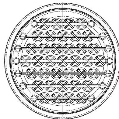
Absorber section with inserted frames of spiral fill Sekce absorberu s vloženými rámy spirálové výplně
