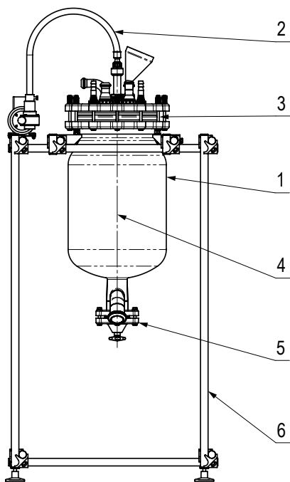
Processing kettle with electric drive and bottom closure Procesní kotlík s elektropohonem a dnovým uzavěrem
