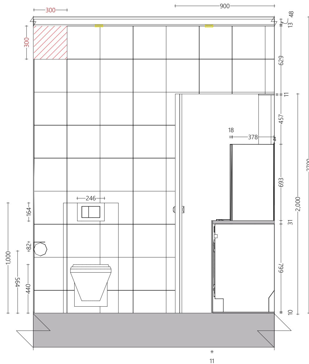
B-B Flisskjema, 1:20
