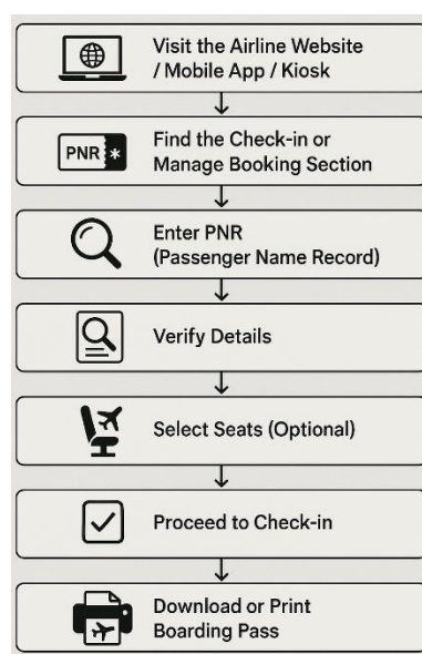
चित्र 1.14 — फ़्लोचार्ट
