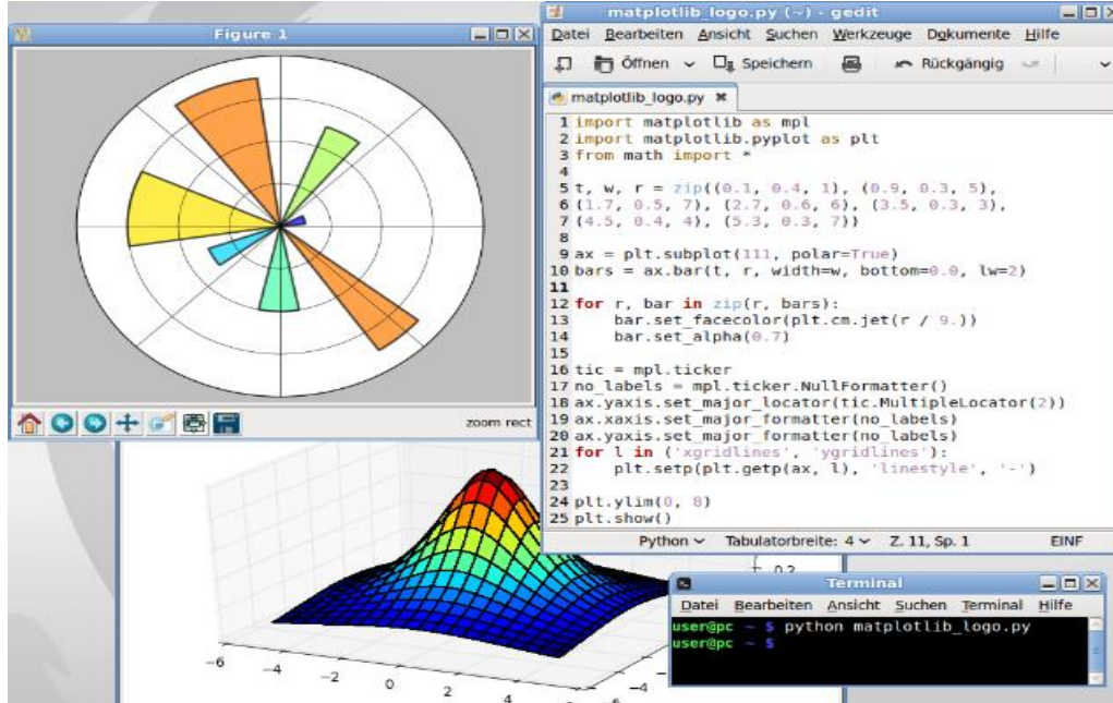
चित्र 2.4— मैटप्लॉटलिब
