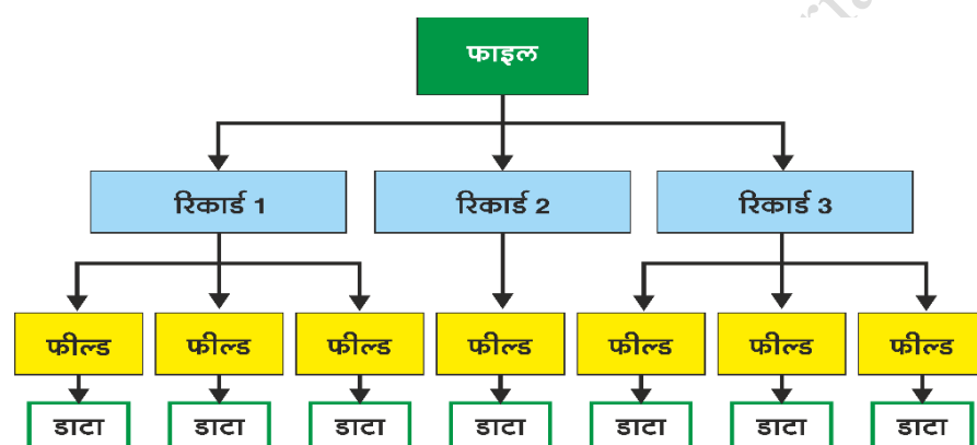
चित्र 1.6— प्राथमिक डेटा संगठन
