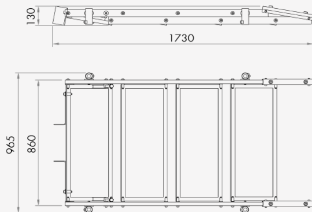
MEDIDAS PLEGADA
