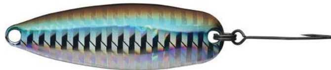
Modèle Coulant Taille (mm) 58 Poids (g) 9 Hameçon 8001 #1SS Qté/Sachet 1
