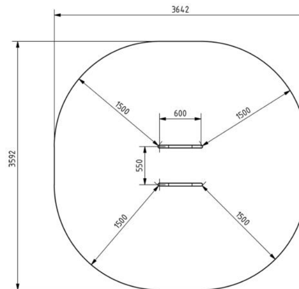
Felülnézet
