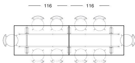
Nr. 5 = Dimensioni piano 330x90
