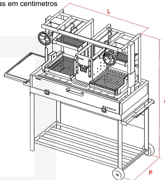
Figura 13 – Dimensões.
