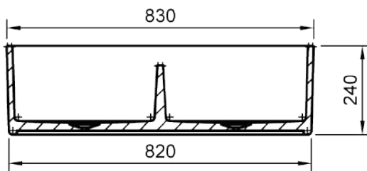
A-A (1:10)
