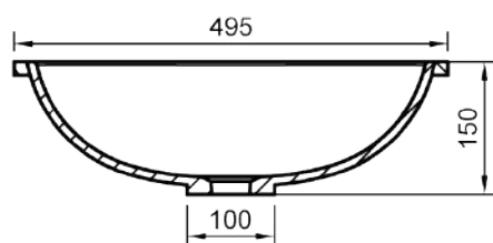
A-A (1:6)
