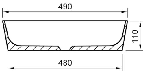
A-A (1:8)
