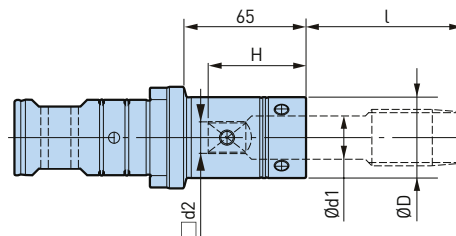
MGT36 (Tap size JIS: M20 - M36; P1/4, P3/4, P1)
