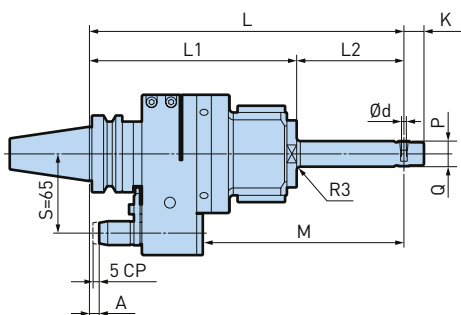
BBT40
